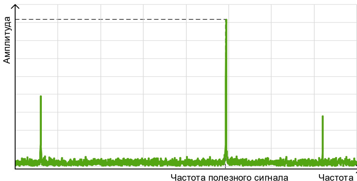
Рисунок 9.4 – Спектр сигнала
